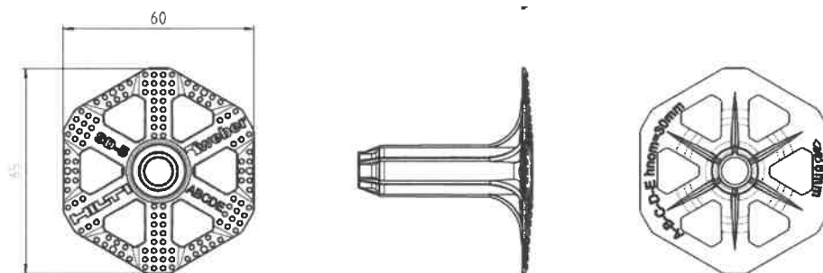
Abbildung A2: Teller
