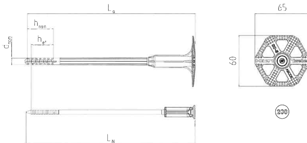
Abbildung A1: Dübelhülse und Dübelteller als Zusammenbau und Kunststoffnagel
